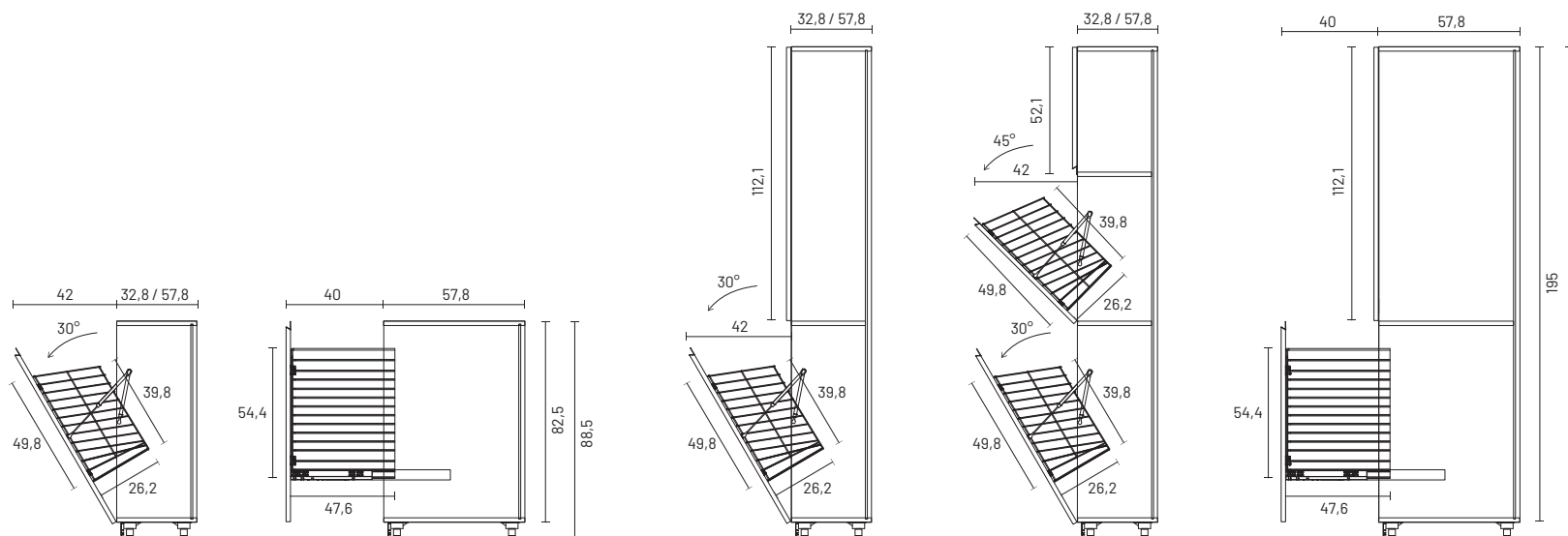
base 1 anta ribalta 1 tilt door base unit
