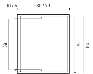
colonna portalavatrice e asciugatrice tall unit for washer and dryer
