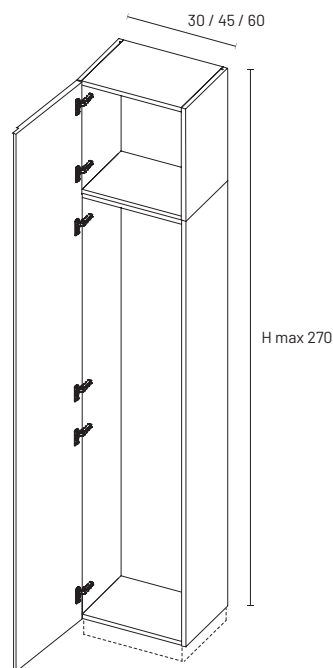
anta dx o sx con maniglia R or L door with handle
