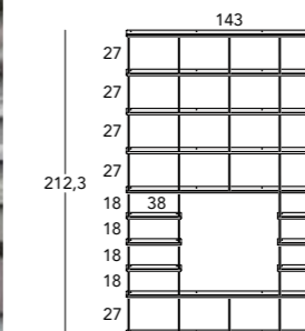
COMP. 07 Laccato antracite/bianco/bronzo € 1.362 L. 143 P. 18,7 H. 212,3 Anthracite lacquer/White/Bronze
