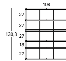
COMP. 19 Laccato antracite/bianco/bronzo € 688 L. 108 P. 18,7 H. 130,8 Anthracite lacquer/White/Bronze
