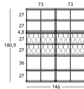
COMP. 20 Laccato antracite/bianco/bronzo € 1.500 L. 146 P. 18,7 H. 180,9 Anthracite lacquer/White/Bronze
