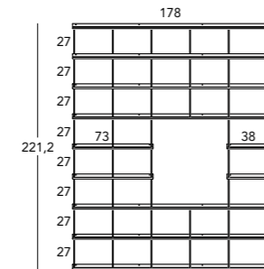
COMP. 02 Laccato antracite/bianco/bronzo € 1.541 L. 178 P. 18,7 H. 221,2 Anthracite lacquer/White/Bronze
