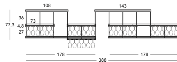
COMP. 21 Laccato antracite/bianco/bronzo € 1.472 L. 388 P. 18,7 H. 77,3 Anthracite lacquer/White/Bronze
